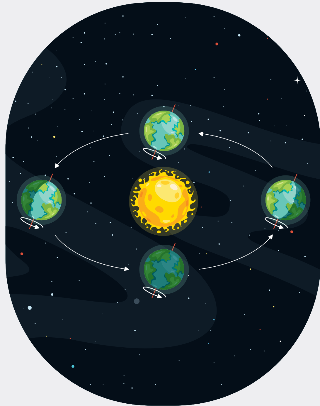
שינוי באנרגיה מהשמש (עונות השנה)
