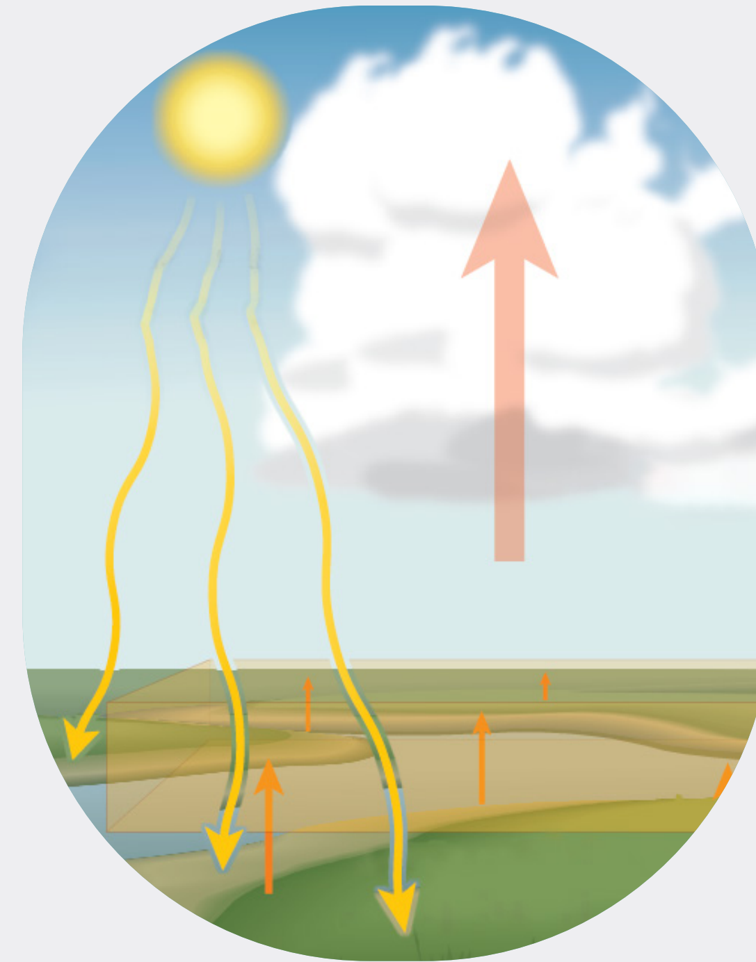
גורמים פנימיים (מעברי אנרגיה)
